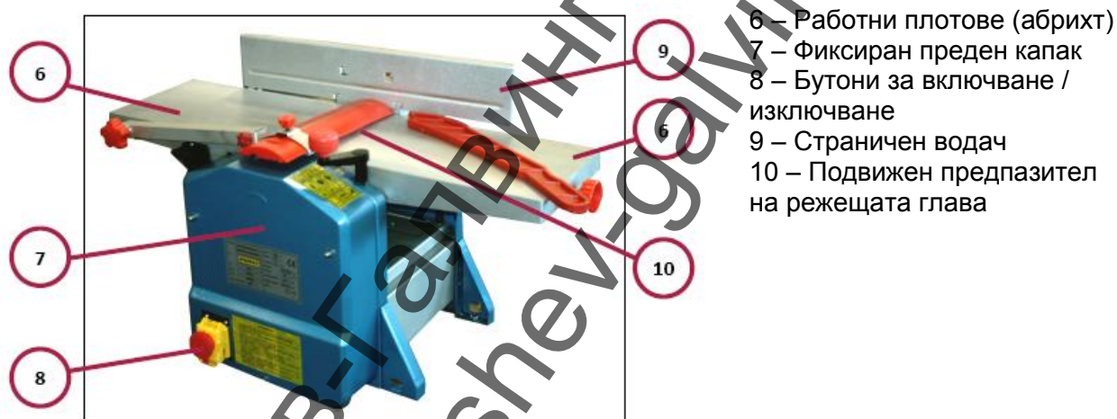
Фигура 1 – Основни части на абрихта – каталожен номер 0686/200
