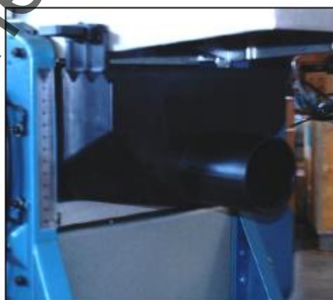
Фигура 20 – Правилно разположение на колектора под работния плот
